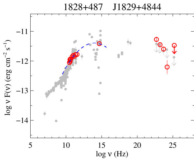
Fig. 98. 1828+487.
