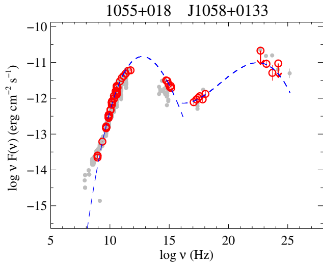
Fig. 67. 1055+018.
