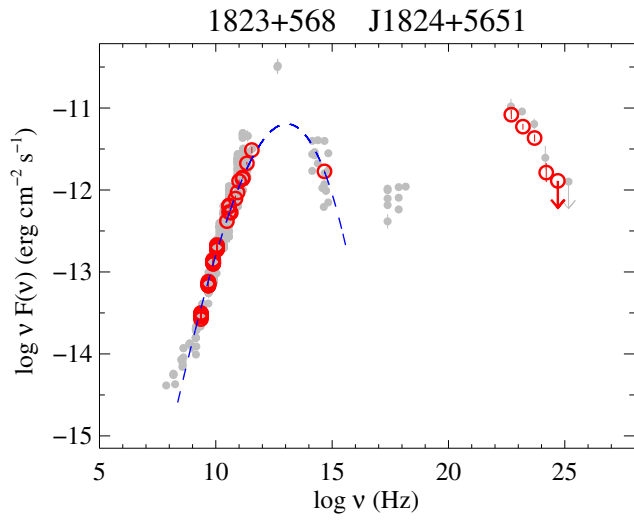
Fig. 97. 1823+568.
