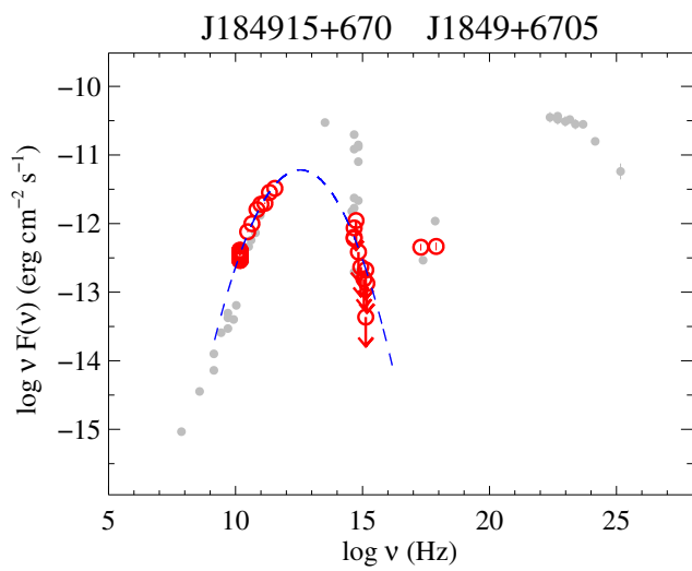
Fig. 99. J184915+670.
