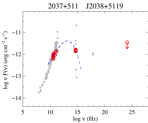
Fig. 105. 2037+511.
