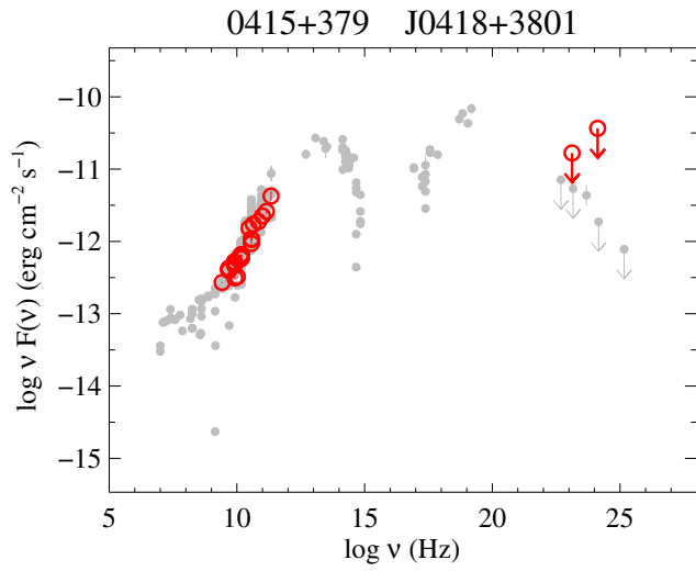
Fig. 37. 0415+379.
