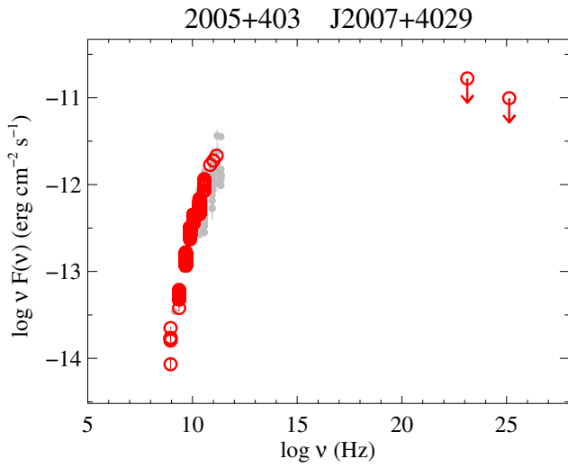
Fig. 103. 2005+403.
