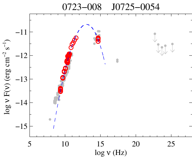
Fig. 48. 0723-008.
