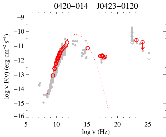
Fig. 38. 0420-014.
