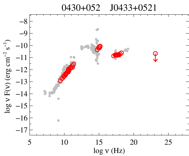
Fig. 39. 0430+052.
