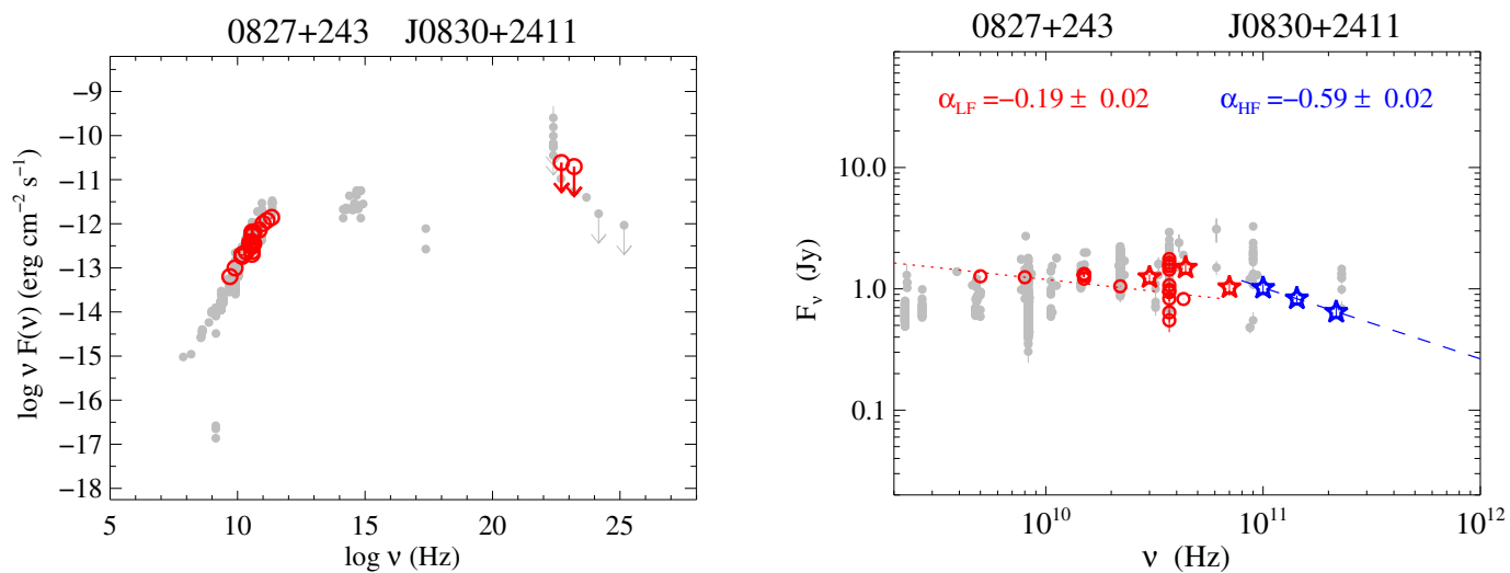
Fig. 56. 0827+243.
