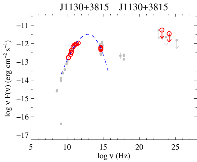
Fig. 68. J1130+3815.
