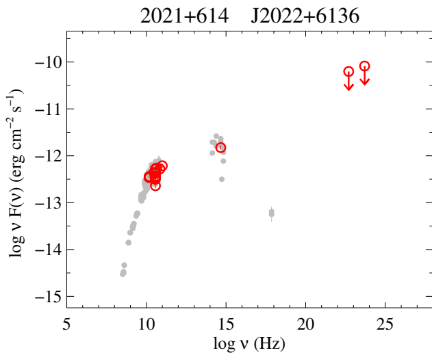
Fig. 104. 2021+614.
