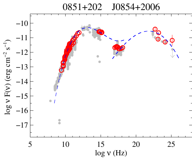
Fig. 58. 0851+202.
