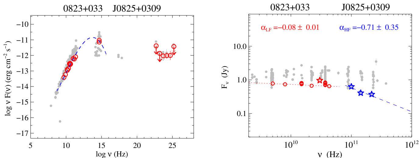
Fig. 55. 0823+033.
