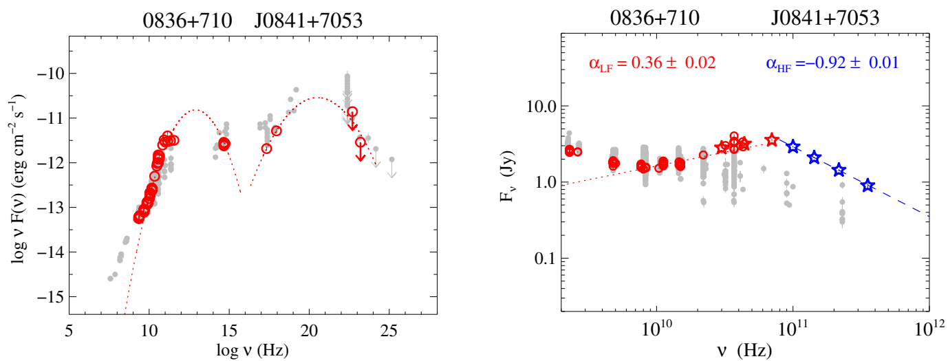
Fig. 57. 0836+710.
