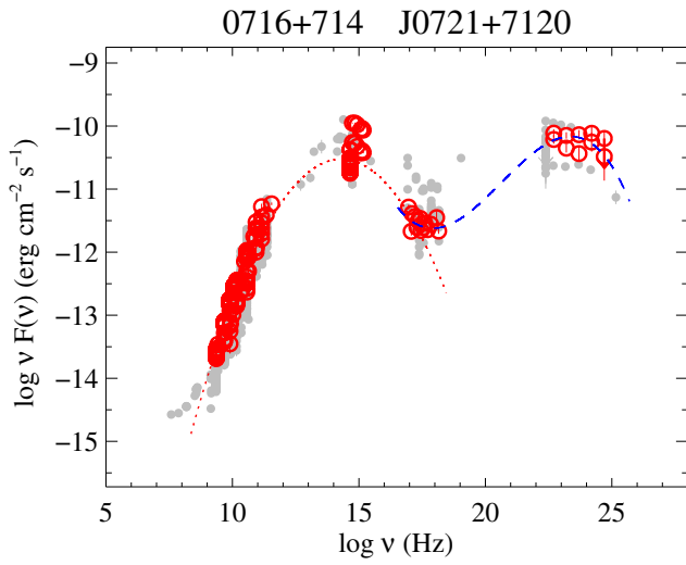
Fig. 47. 0716+714.
